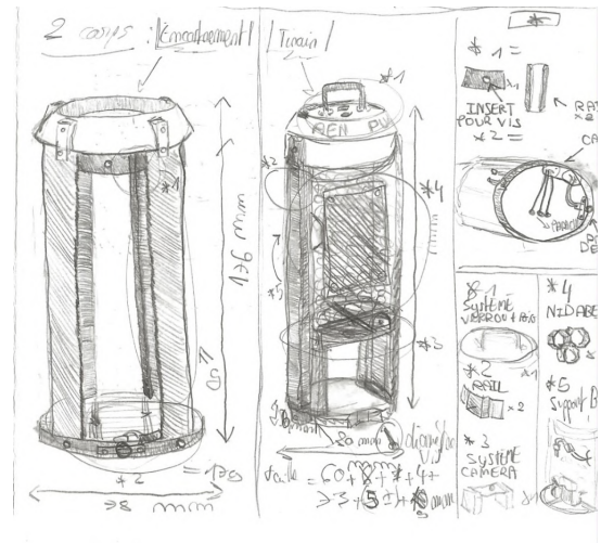
Figure 14 : premiers croquis de la partie “tiroir”.
