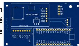
Figure 2 : Première version de l'ordinateur
