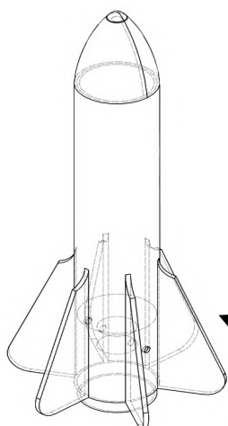
Figure 3 : Notre premier modèle 3D de fusée et le logo associé au projet « Nova 01 tiny » (voir Annexe 2 pour une photo de la fusée).
