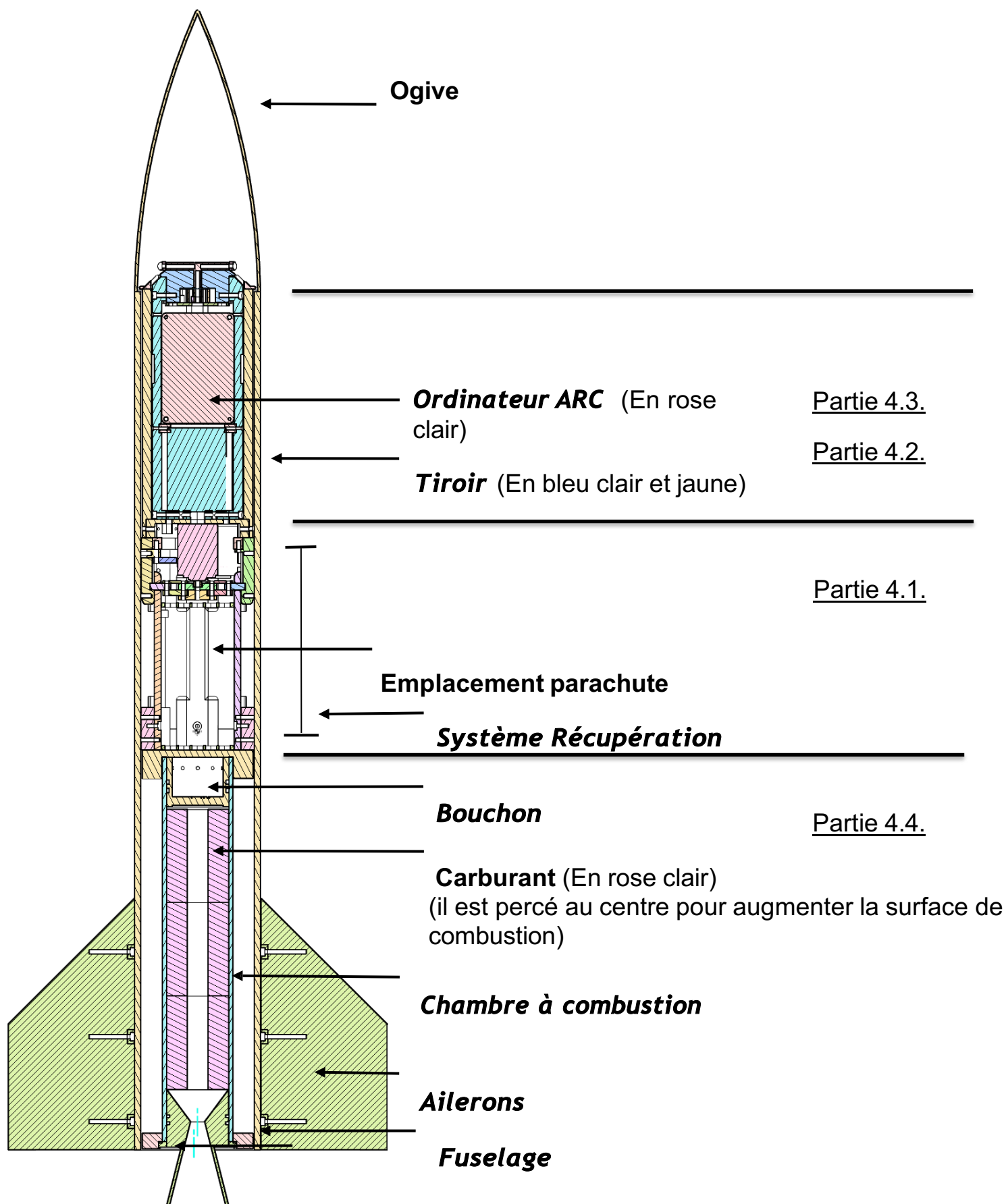
Figure 6 : Schéma complet de la fusée.
